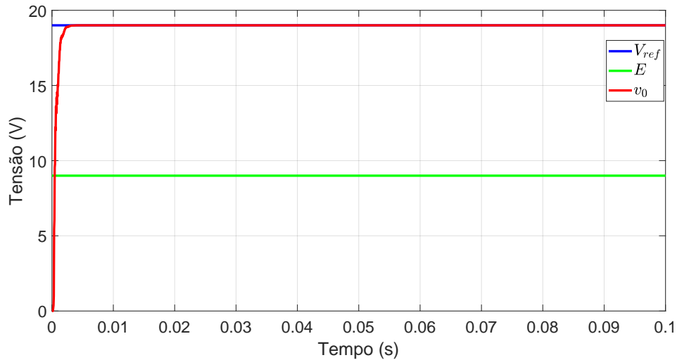
Figura 4: Resposta do sistema em malha fechada com controlador deadbeat operando sem surtos.
