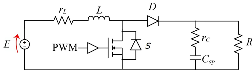
Figura 1: Circuito elétrico do conversor boost.
