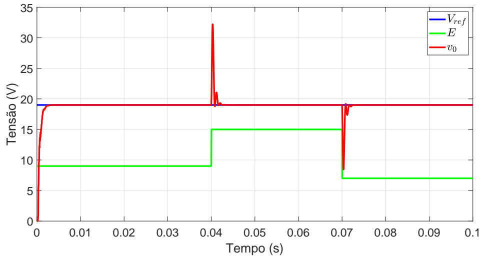
Figura 6: Resposta do sistema em malha fechada com controlador deadbeat operando com surtos.
