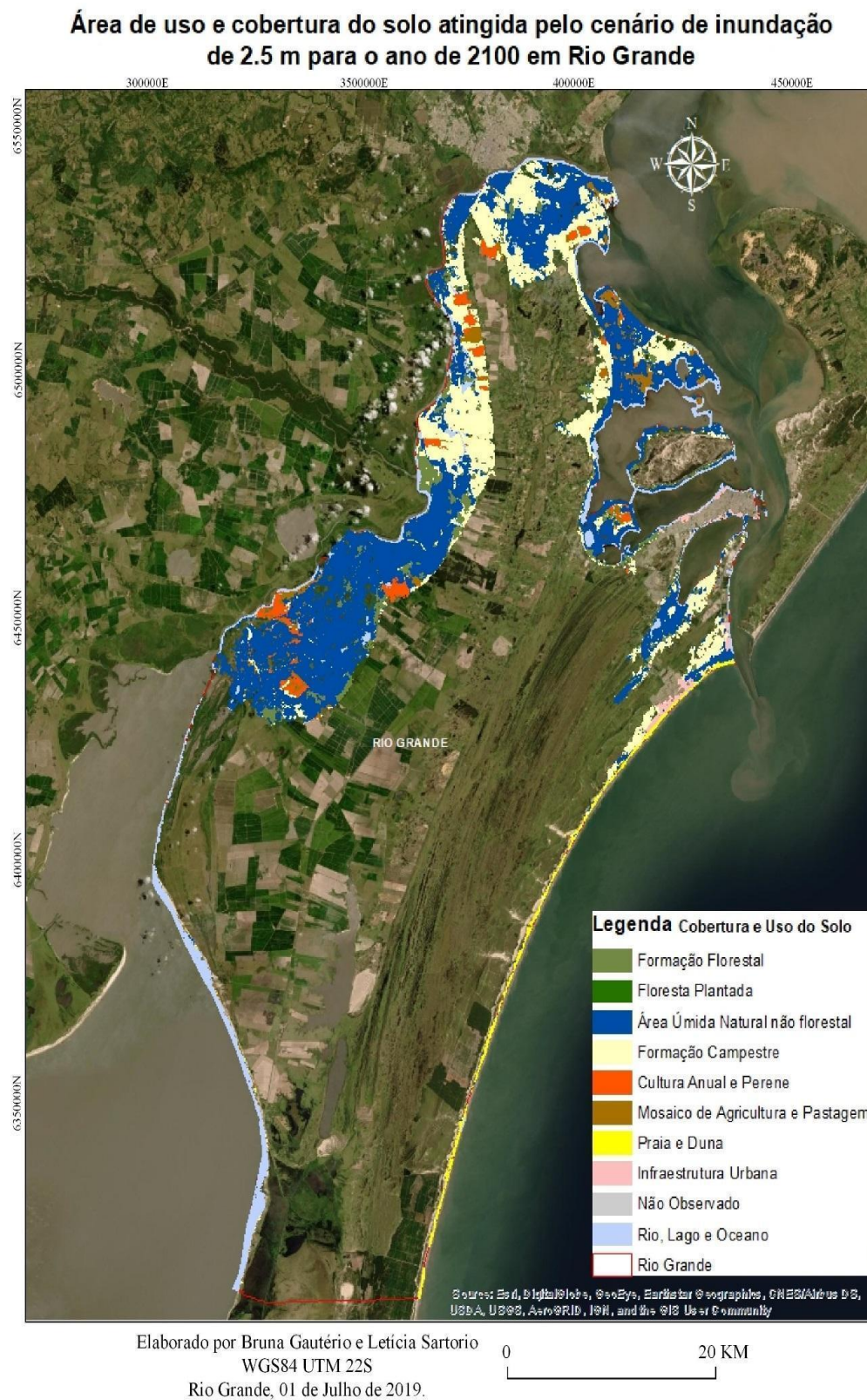
Figura 2: Área de uso e cobertura do solo atingida pelo cenário de inundação de 2.5 m para o ano de 2100 em Rio Grande - RS.
