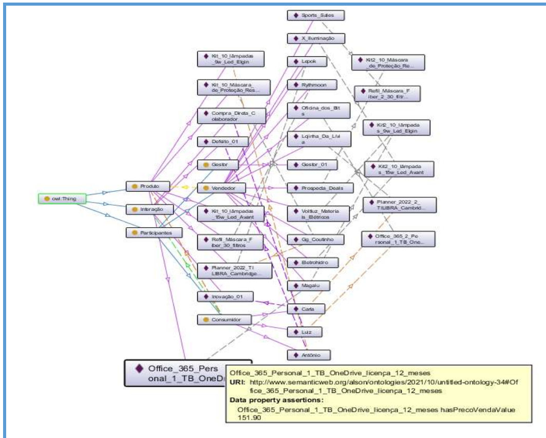
Figura 5 – Grafo da relação entre indivíduos e classes – caso “Alfa”
